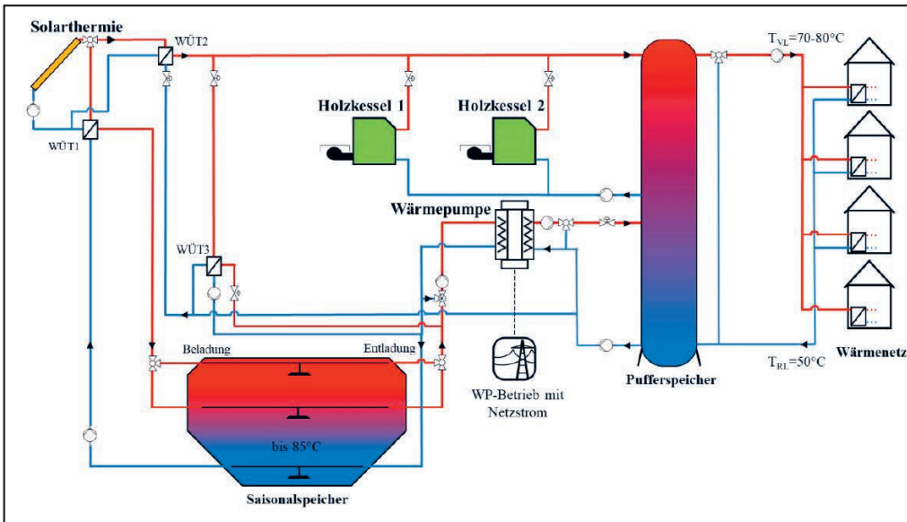
Schematische Darstellung der Solarwärme in Bracht (Skizze: Universität Kassel)
