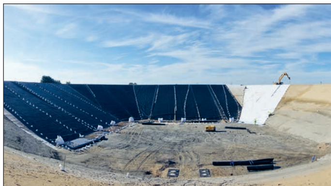
Meldorf, Schleswig-Holstein. Speicherbecken mit 45.000 m 3 Volumen im Bau. Links fertige Auskleidung, das weiße Vlies rechts hinten gehört zur Unterkonstruktion.
