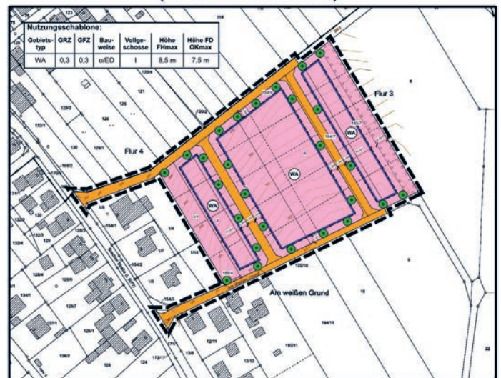
Räumlicher Geltungsbereich und Entwurf des Bebauungsplans "Am weißen Grund" (Planteil - unmaßstäblich)
